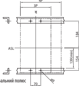
Розмітка монтажних отворів
