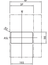
Вирізи в панелі (вигляд спереду)
