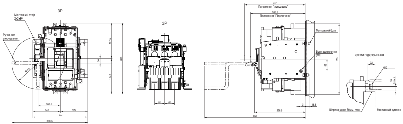
EB2 400 D/O
