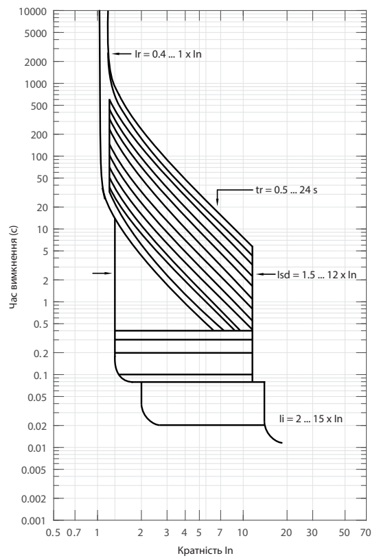
NBS-E&EC LCD (100 - 630A) Характеристика t-I
