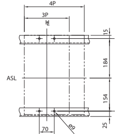
Розмітка монтажних отворів
