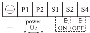
Схема підключення мотор-приводу
