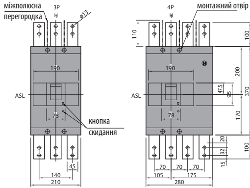
Фронтальне підключення
