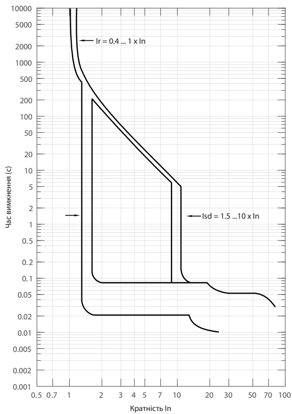
NBS-E (100 - 630A) Характеристика t-I
