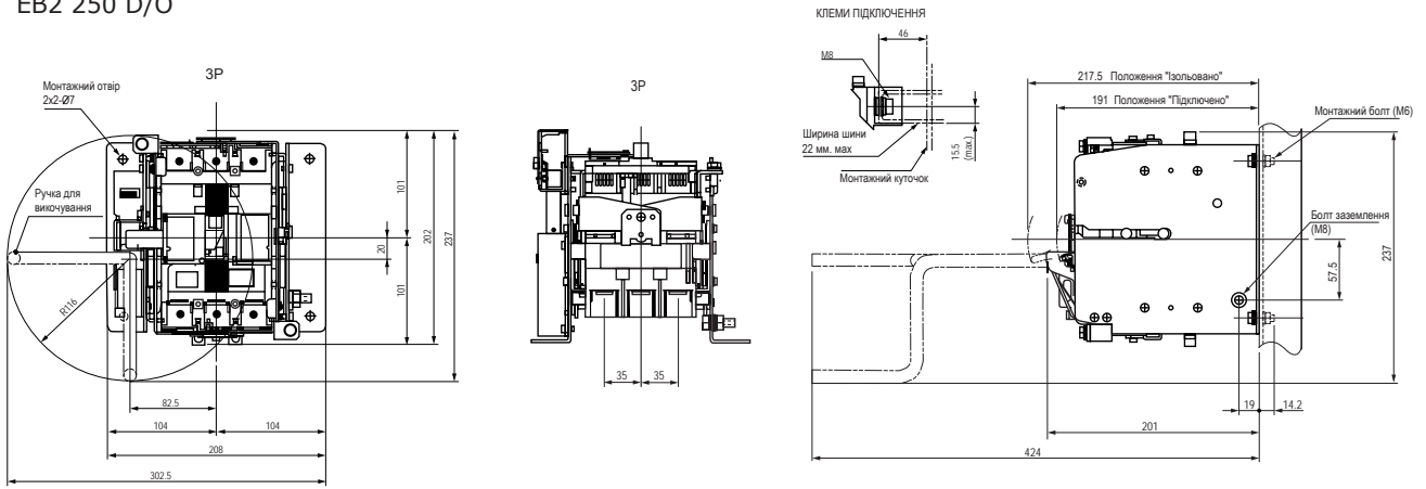
EB2 250 D/O
