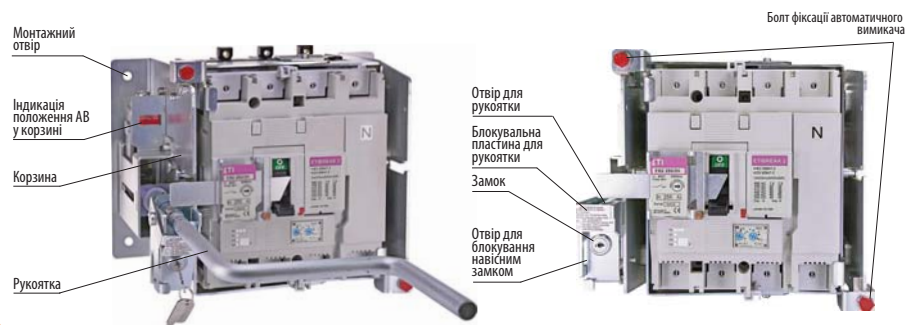
З'єдн. блок DOCK + АВ
