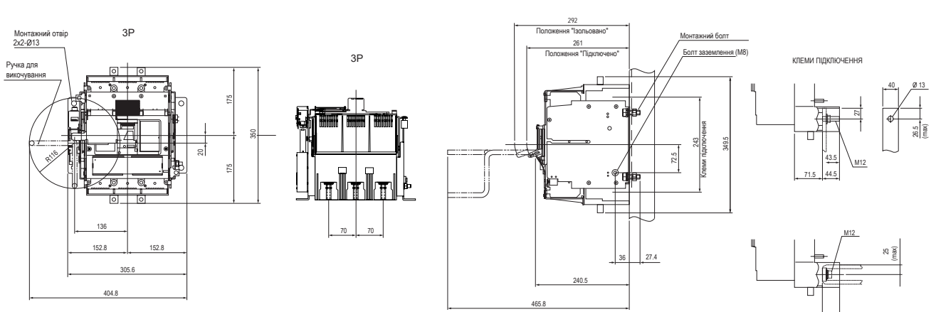
EB2 800 D/O
