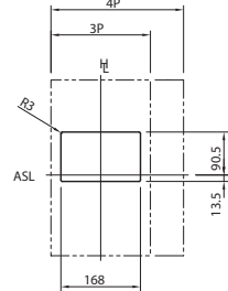
Вирізи в панелі (вигляд спереду)
