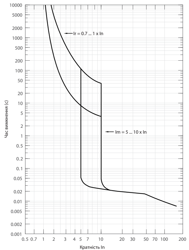
NBS-TMD 400/3 (315, 400A) Характеристика t-I
