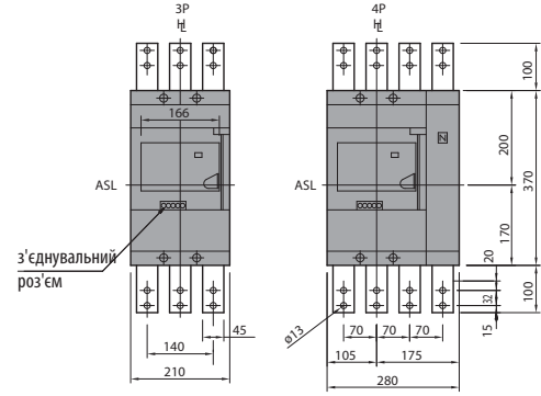
Заднє підключення з мотор-приводом
