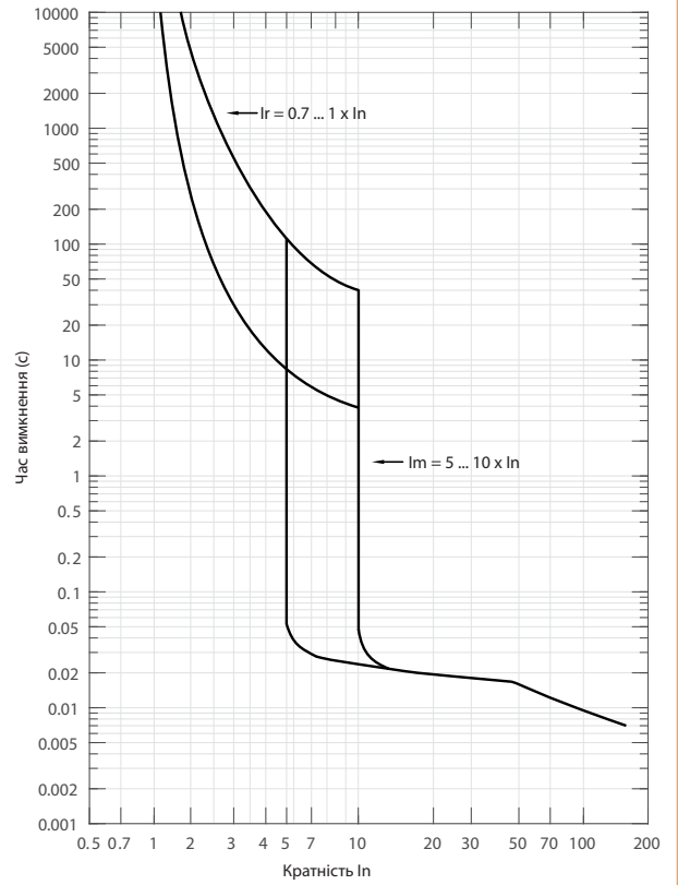
NBS-TMD 630/3 (500, 600A) Характеристика t-I
