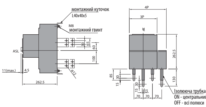
Заднє підключення з мотор-приводом
