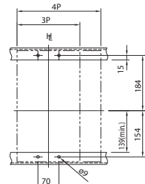
Розмітка монтажних отворів
